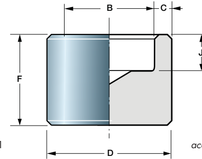
Emboîtement à souder suivant ASME B 16-11 - 1991
